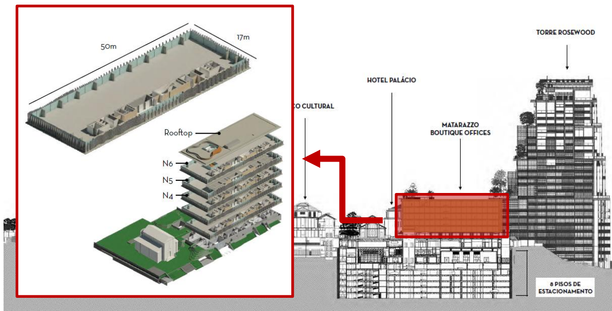
Matarazzo Boutique Offices – Corte das construções e Detalhe das unidades
